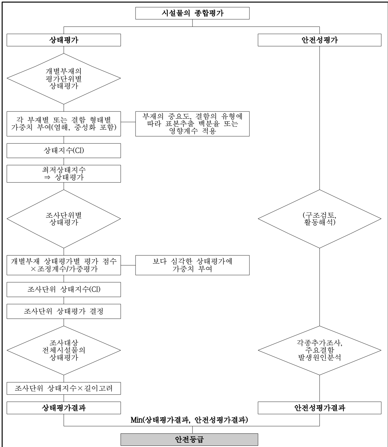
【그림 I -5.1】 종합평가 결과의 산정 흐름도
